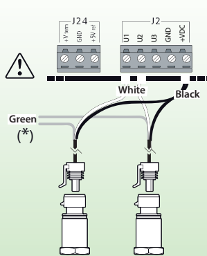
4-20 mA Probe:
